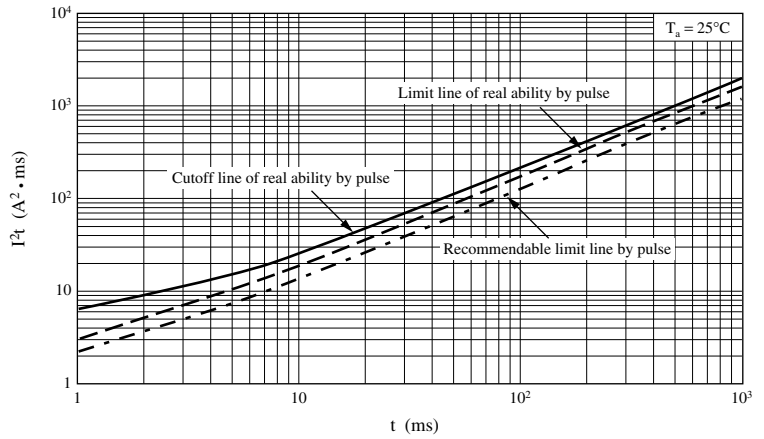
I^2t — t
