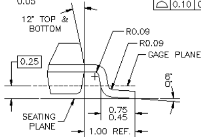
DETAIL A SCALE: 2X
