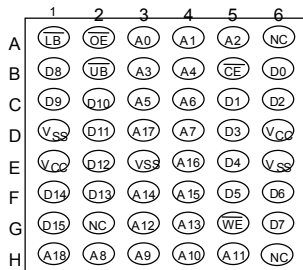
48-Ball CSP top View
