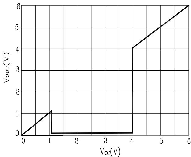
Fig. 1 V_{OUT} - V_{CC}
