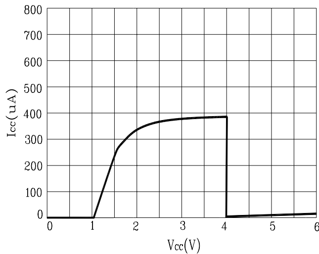
Fig. 2 I_{CC} - V_{CC}
